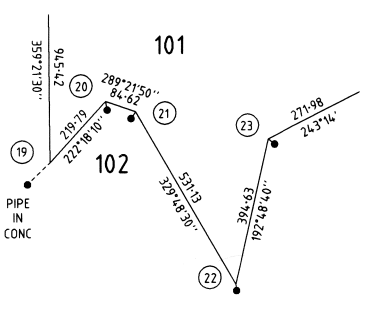
Enlargement E3 NOT TO SCALE
