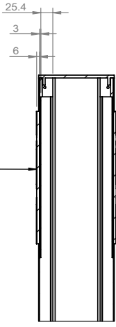
SECTION R-R SCALE 1 : 10
